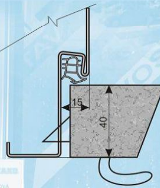
Tvar polodrážky v zárubni - pro dveře bezpolodrážkové
