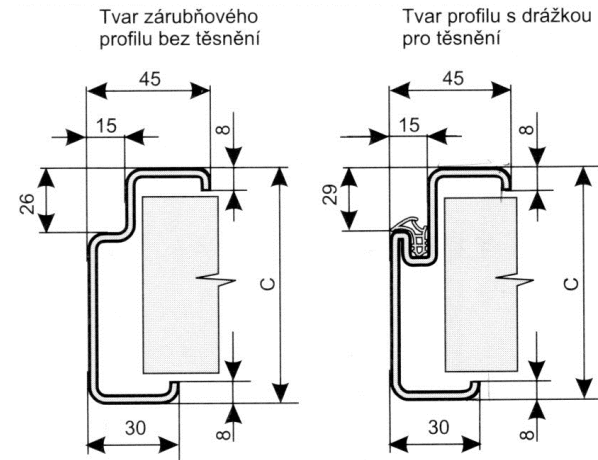
profil H (klasické zdění)
