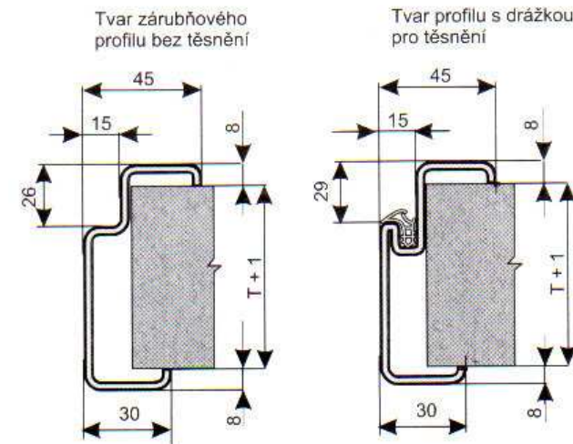
profil YH (přesné zdění)
