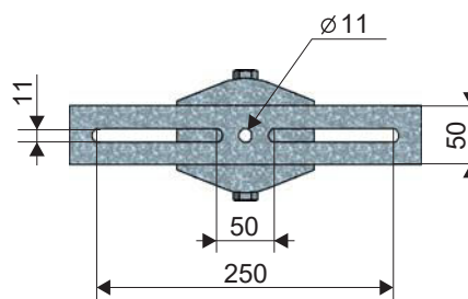
Otvory pro uchycení reflektoru URA
